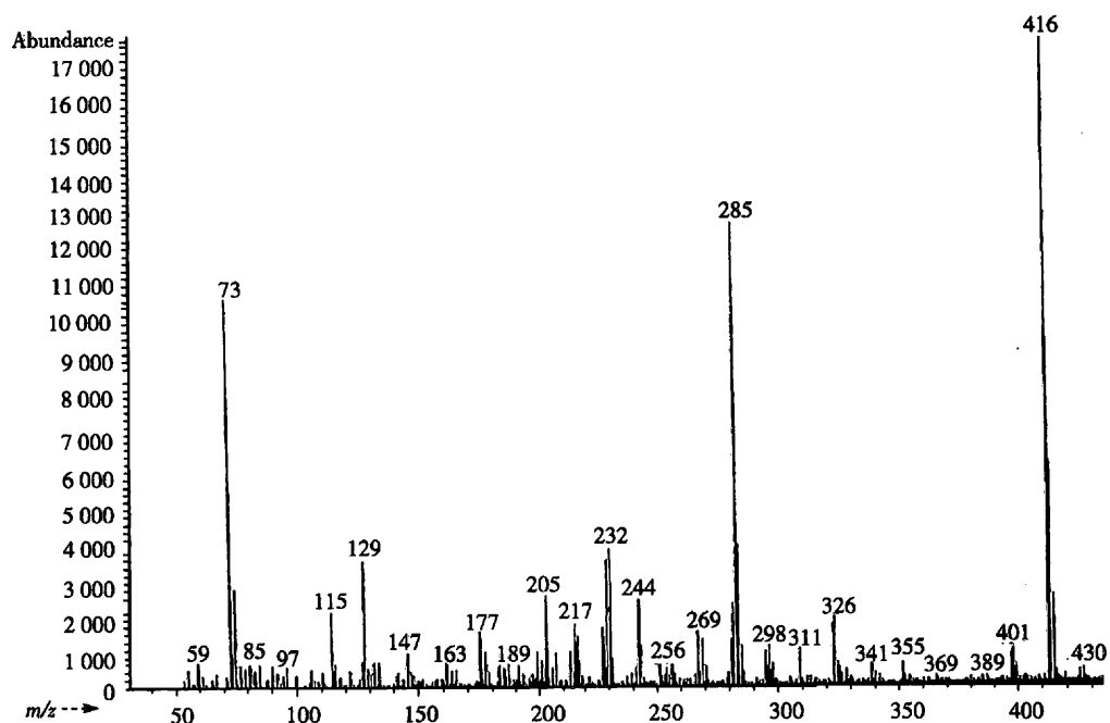
图 A.1 \beta -雌二醇全扫描质谱图 (特征离子 m/z : 416, 326, 285, 232; 定量离子 m/z : 416)
