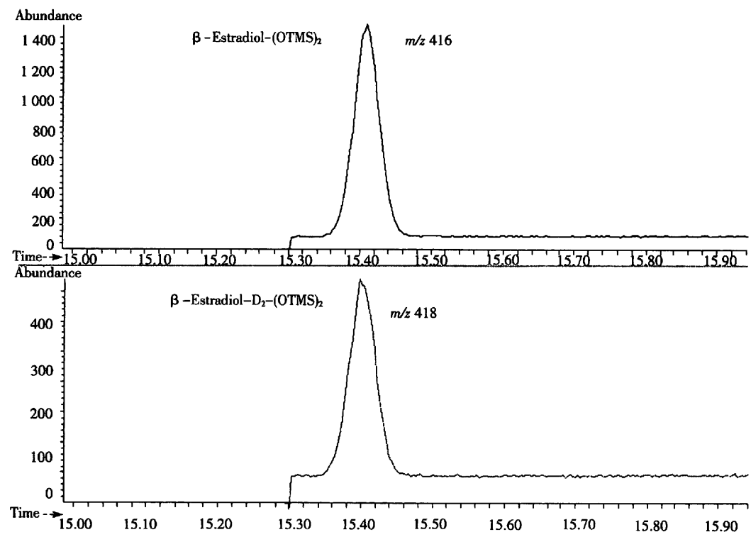
图 A. 3 \beta -雌二醇(0. 25 \mu\text{g}/\text{mL} )与 \beta -雌二醇- D 2 标准溶液(0. 05 \mu\text{g}/\text{mL} )衍生物的定量离子的质量色谱图
