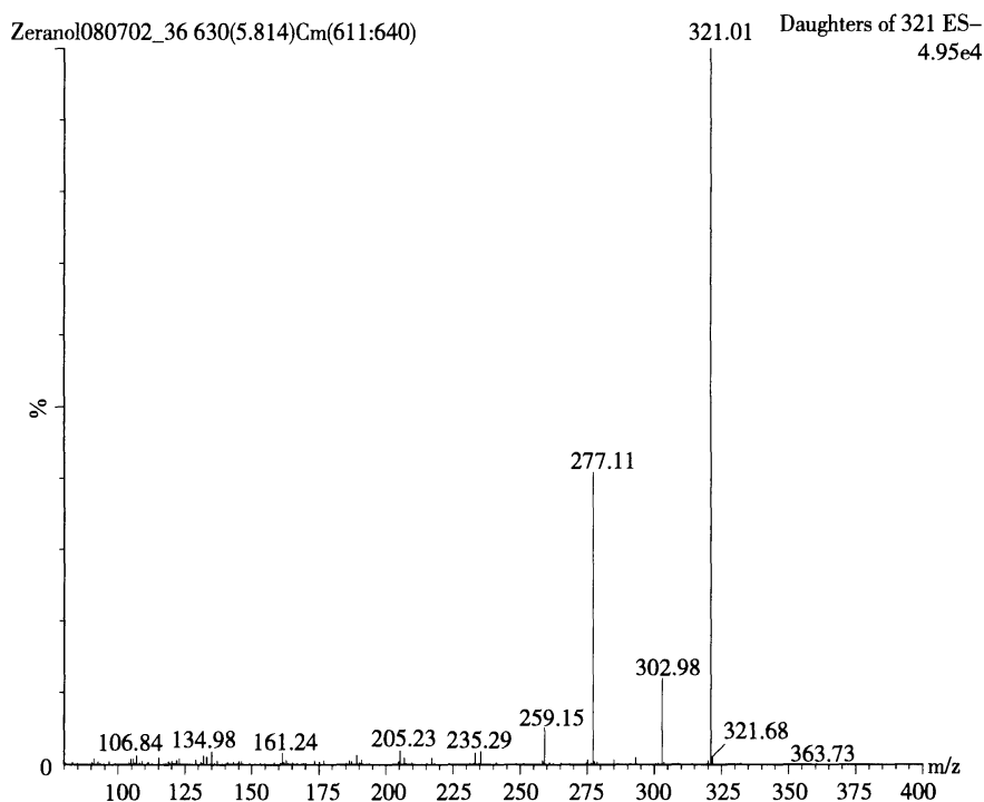
图 A.2 \beta -玉米赤霉醇与 \alpha -玉米赤霉醇子离子扫描质谱图
