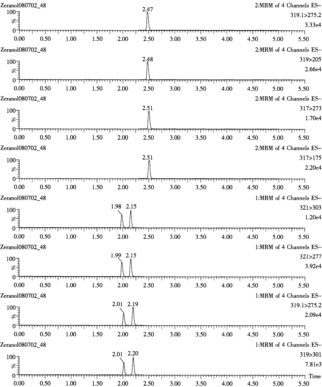
图 A.1 玉米赤霉醇类标准溶液特征离子质量色谱图
