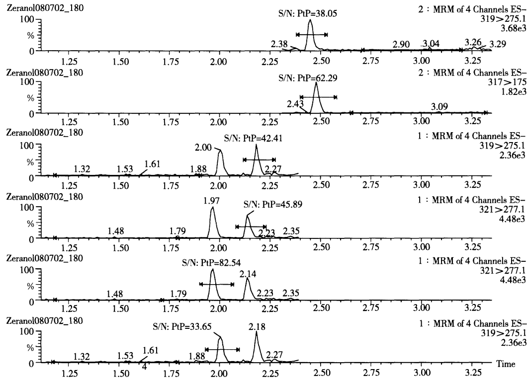
图 A. 6 基质(鱼)加标回收率色谱图(0.5 \mu\text{g/kg} )
