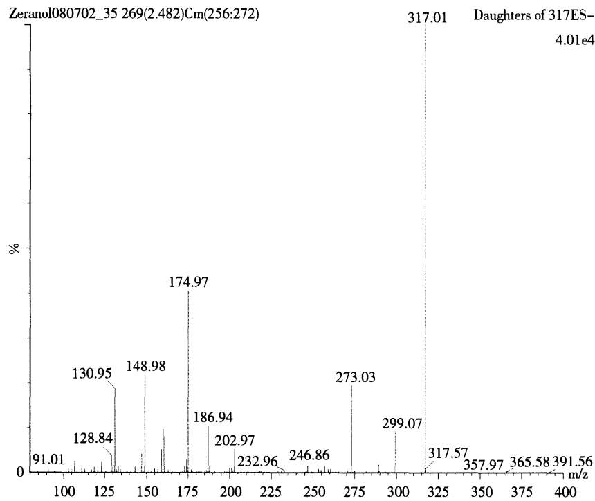
图 A. 4 玉米赤霉酮子离子扫描质谱图
