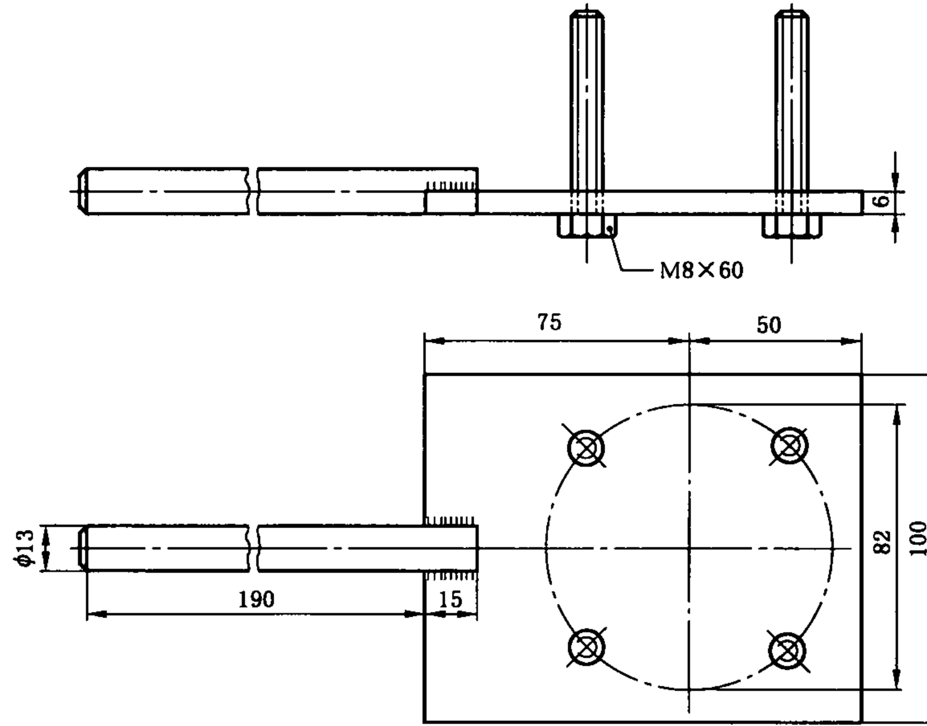
图 7 试验槽支架
