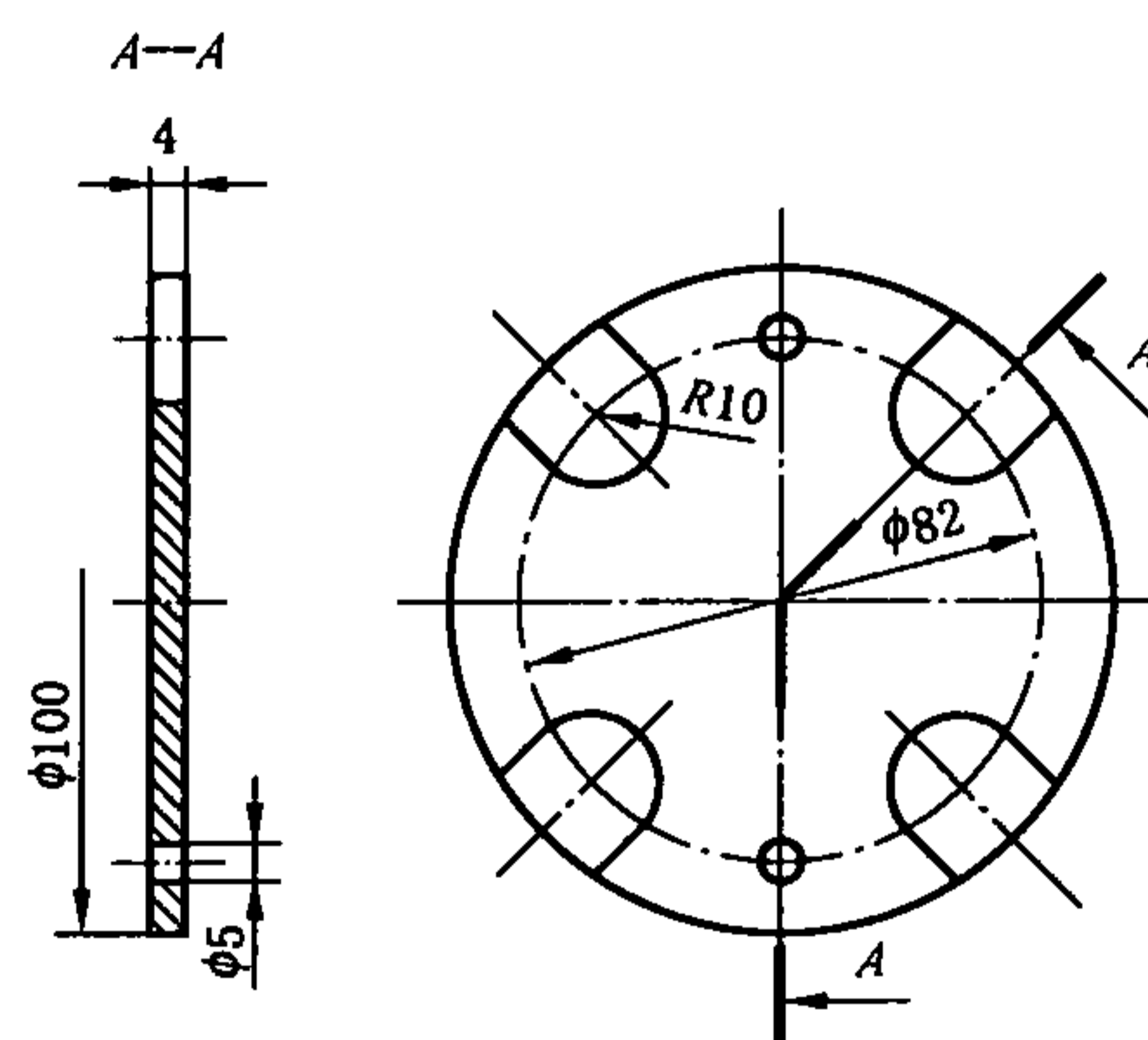
图 10 透明盖(可选)
