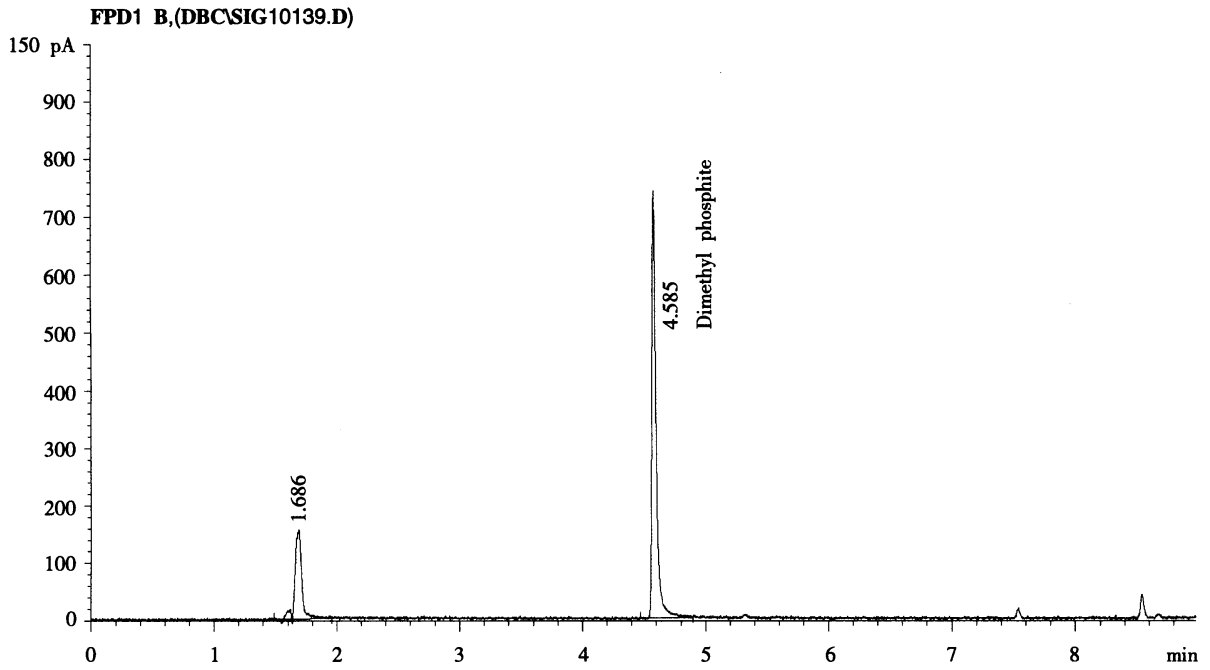
图 A.1 敌百虫分解产物亚磷酸二甲酯色谱图
